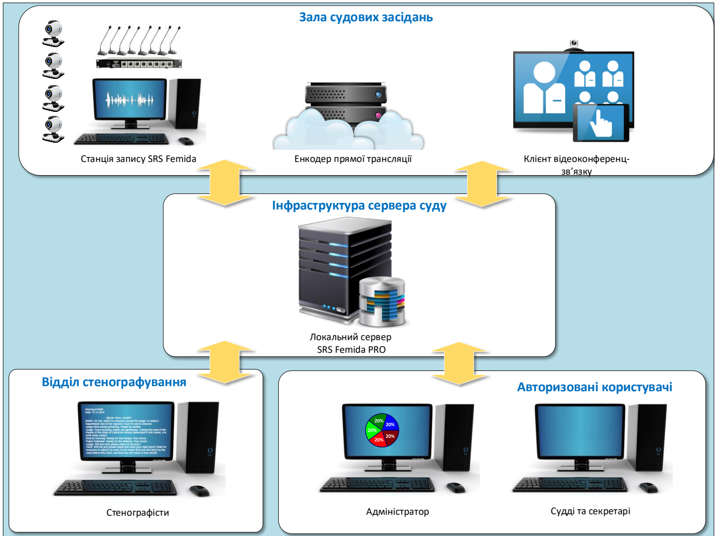
Архітектура системи "SRS Femida Pro"
